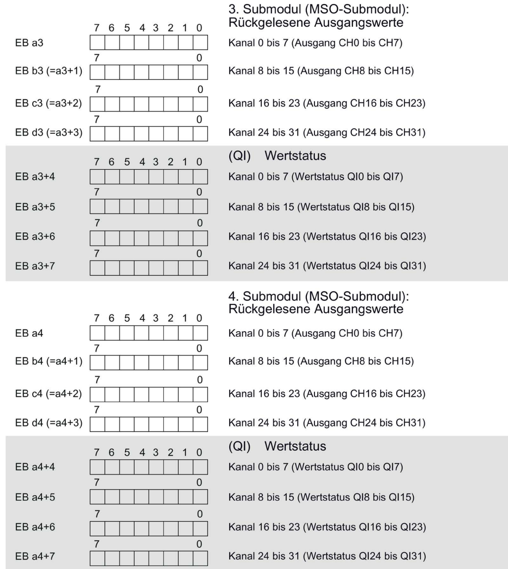
Bild 4-4 Adressraum bei Konfiguration als 1 x 32-kanaliges DQ 32x24VDC/0.5A HF S MSO mit Wertstatus
